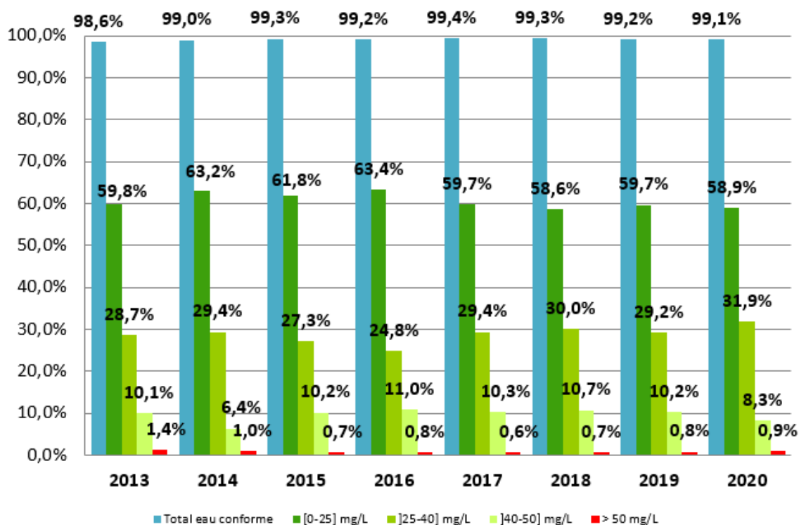
Figure 2 : Evolution de la répartition de la population en fonction de la concentration maximale annuelle en nitrates entre 2013 et 2020
